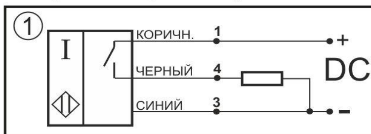
Нормально-разомкнутый контакт
