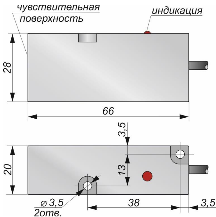
Габаритный чертеж
