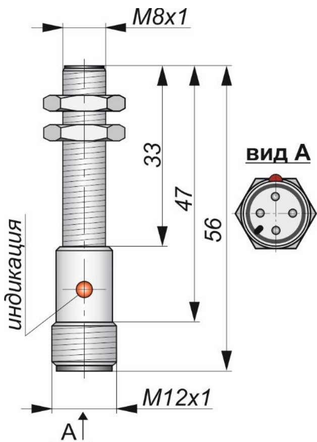
Габаритный чертеж
